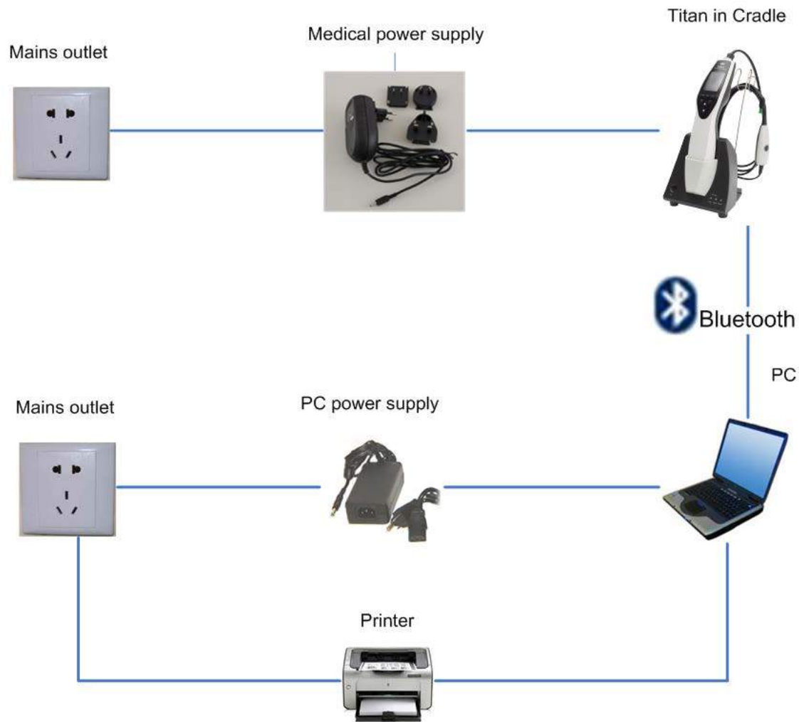
Fig. 5. Titan gebruikt met de cradle, medisch goedgekeurde netvoeding en Bluetooth-aansluiting op de computer
