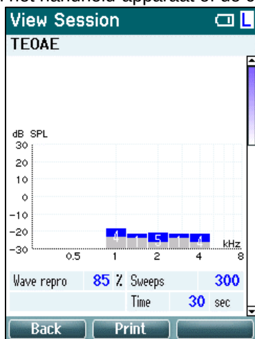
Afbeelding 1 - Probetest is geslaagd/functionerende probe
