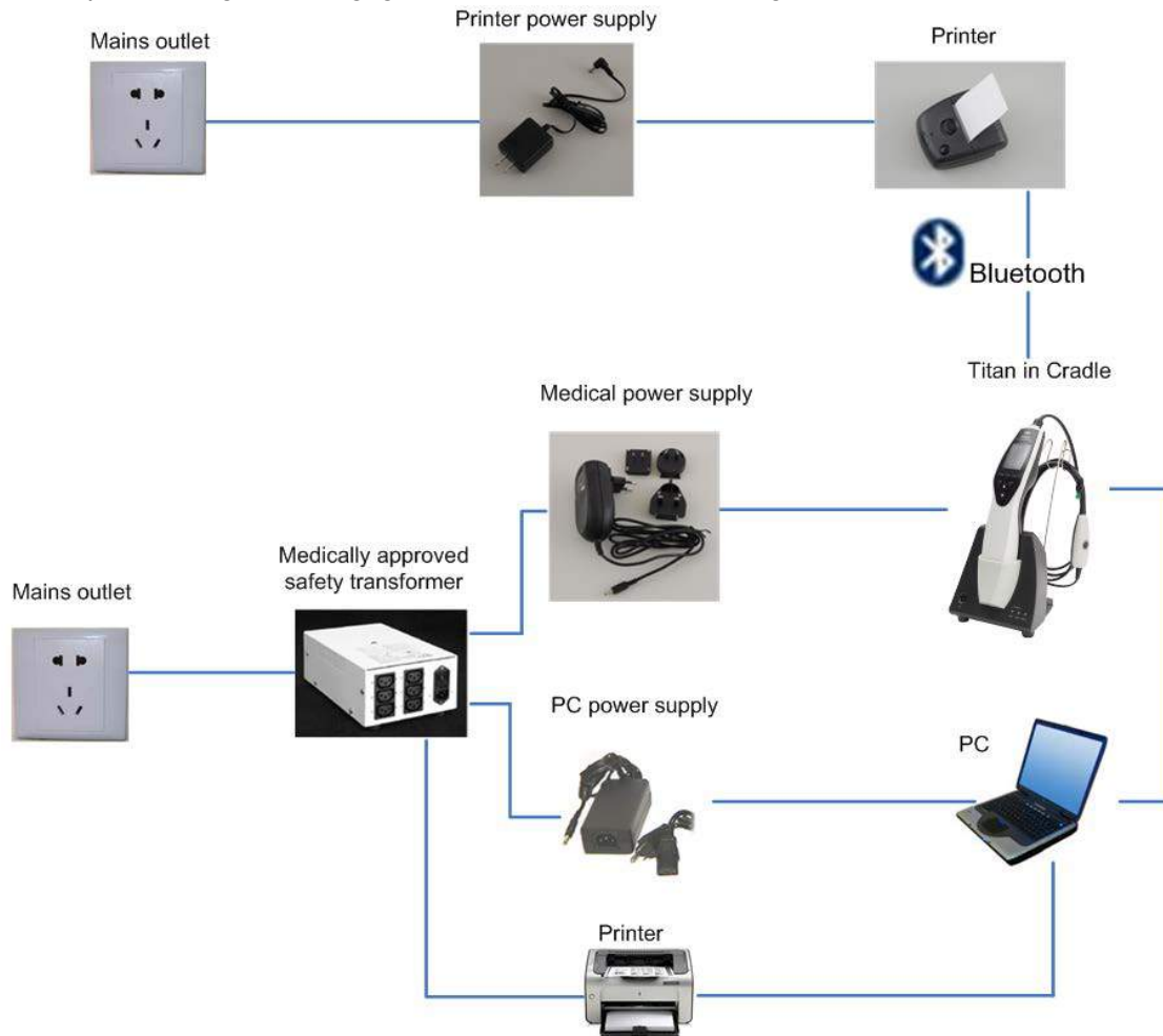
Fig. 7. Titan gebruikt met de cradle, medisch goedgekeurde transformator, een bedrade aansluiting op de computer en een Bluetooth-aansluiting op de printer. Niet geschikt voor gebruik met ABRIS440 omdat patiëntveiligheid niet gegarandeerd kan worden - zie Fig. 8.
