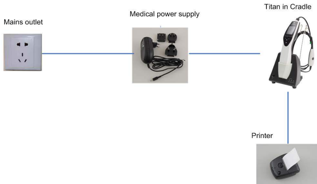
Fig. 4. Titan gebruikt met de cradle, medisch goedgekeurde netvoeding en een bedrade printer gevoed door een batterij
